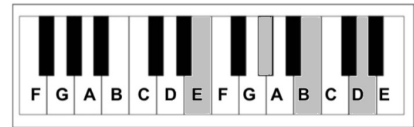
E7: E-G#-B-D
