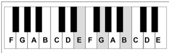
Em: E-G-B
