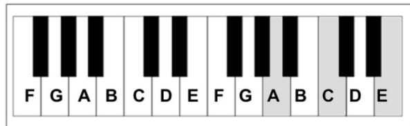
Am: A-C-E
