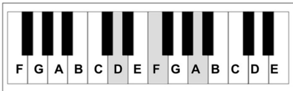
Dm: D-F-A
