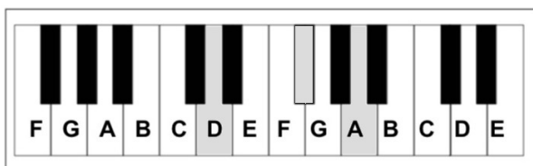
D Major: D-F#-A
