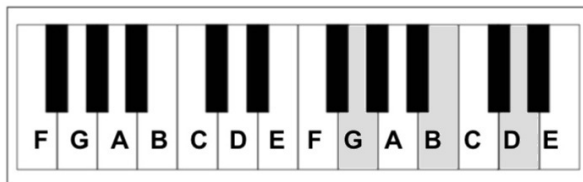
G Major: G-B-D
