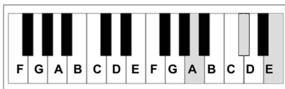
A Major: A-C#-E
